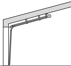
Beschlag LD mit Dachfolge
