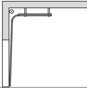
Beschlagsart H Höhergeführter Laufschienen-Beschlag
