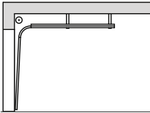
Beschlagsart N Normal-Beschlag
